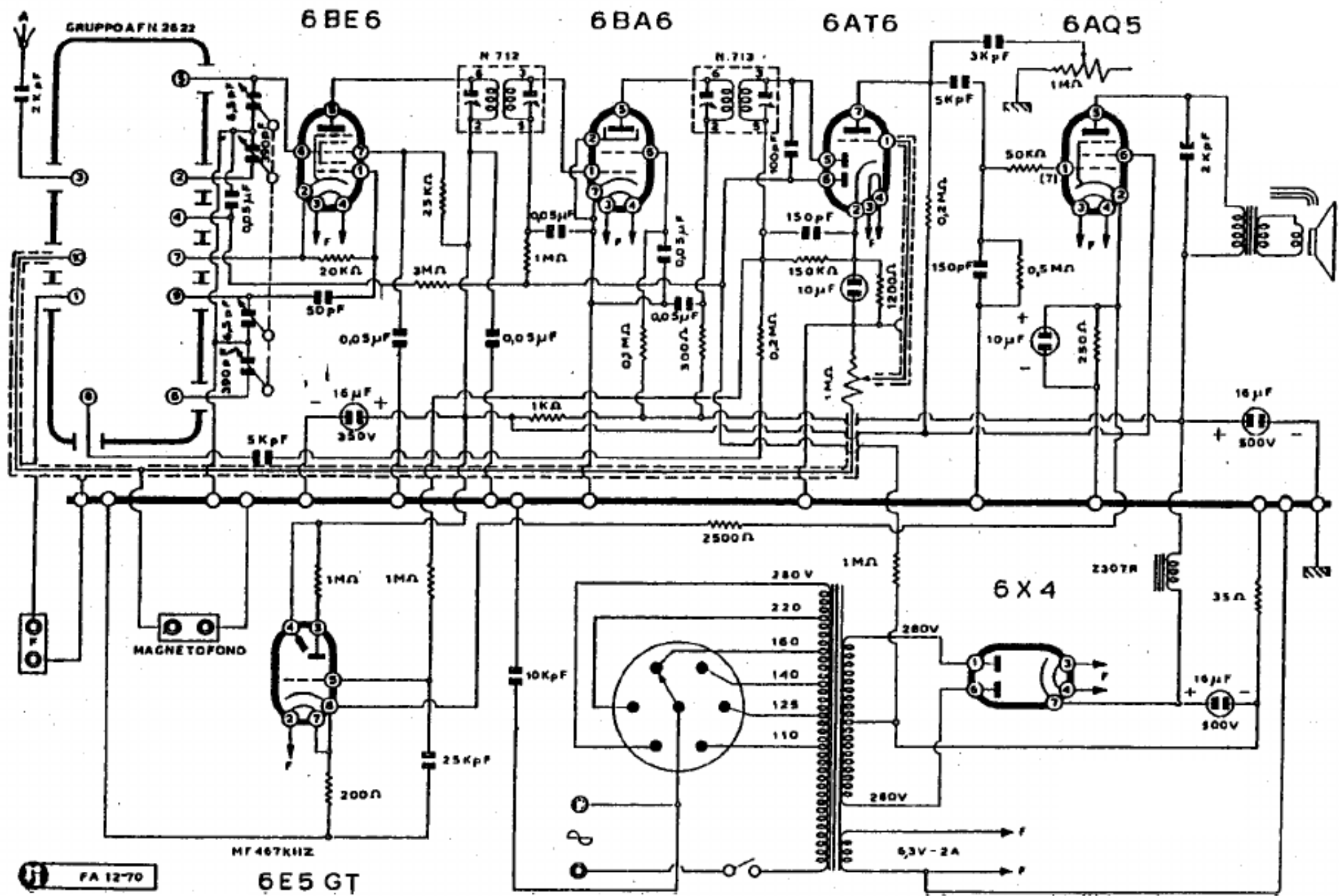
GELOSO S.A. - Mod. Super G 133
